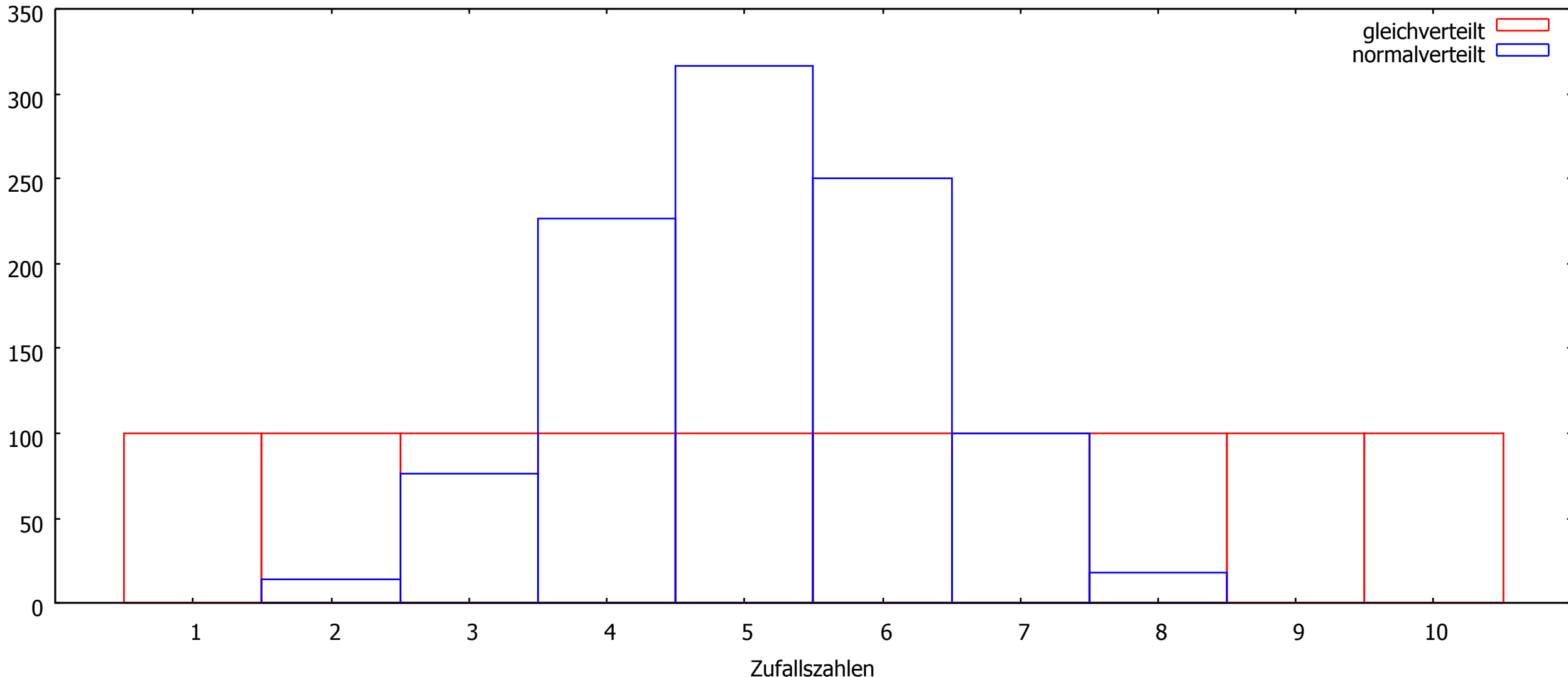
Vergleich Gleich- und Normalverteilung
